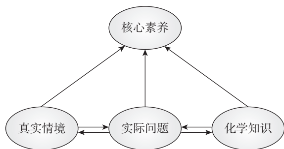
图4 命题框架
